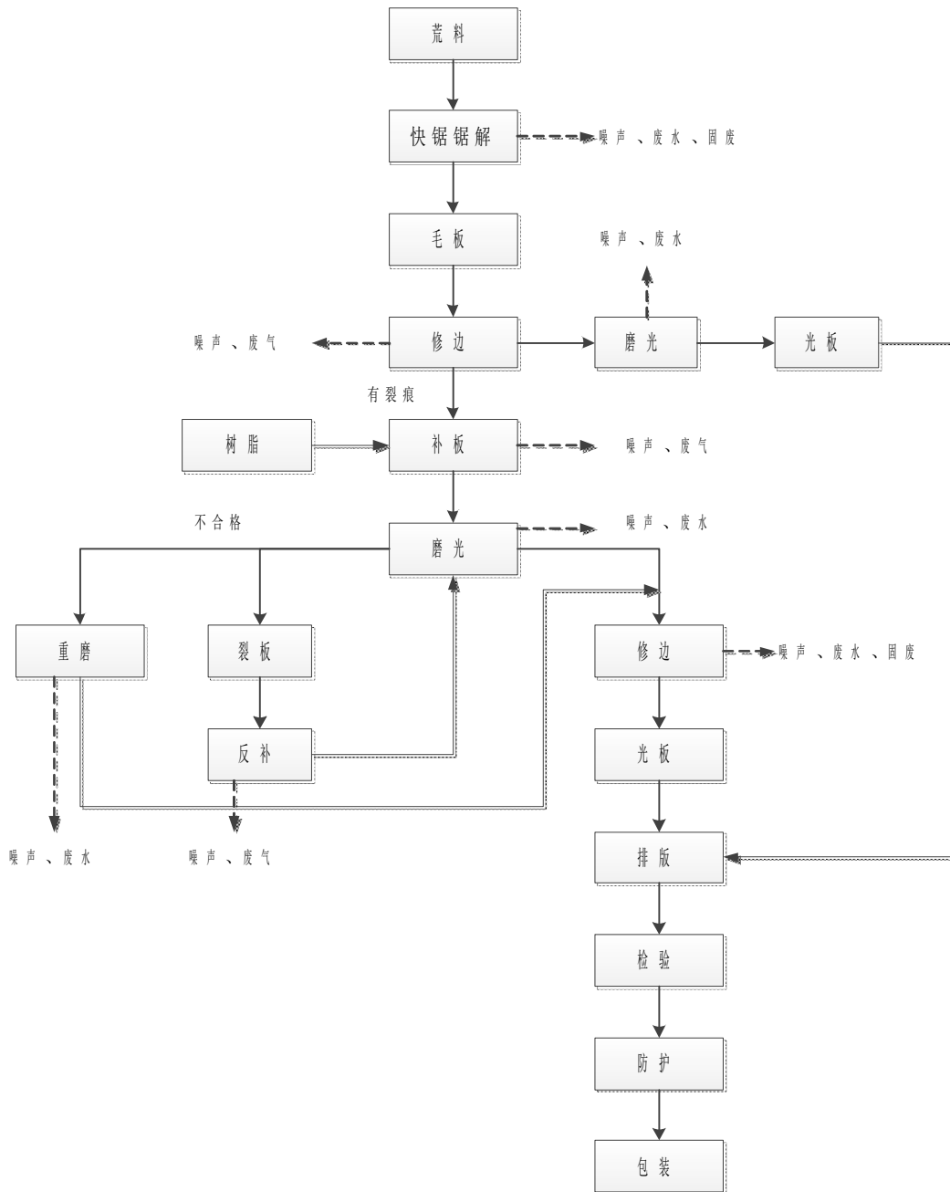
图 4.2-1 天然石材生产工艺
