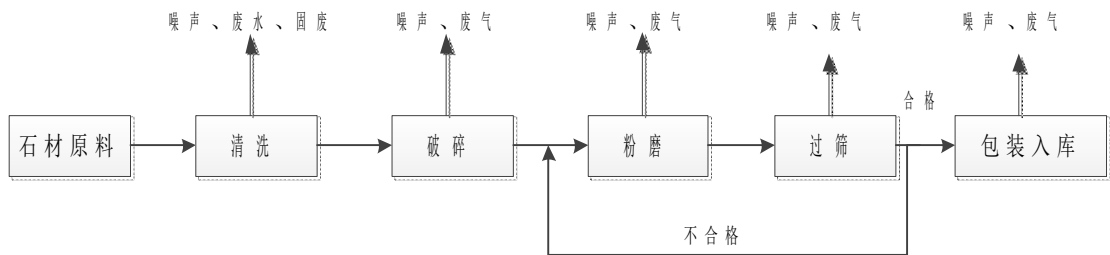
图 4.3-2 复粉生产工艺
