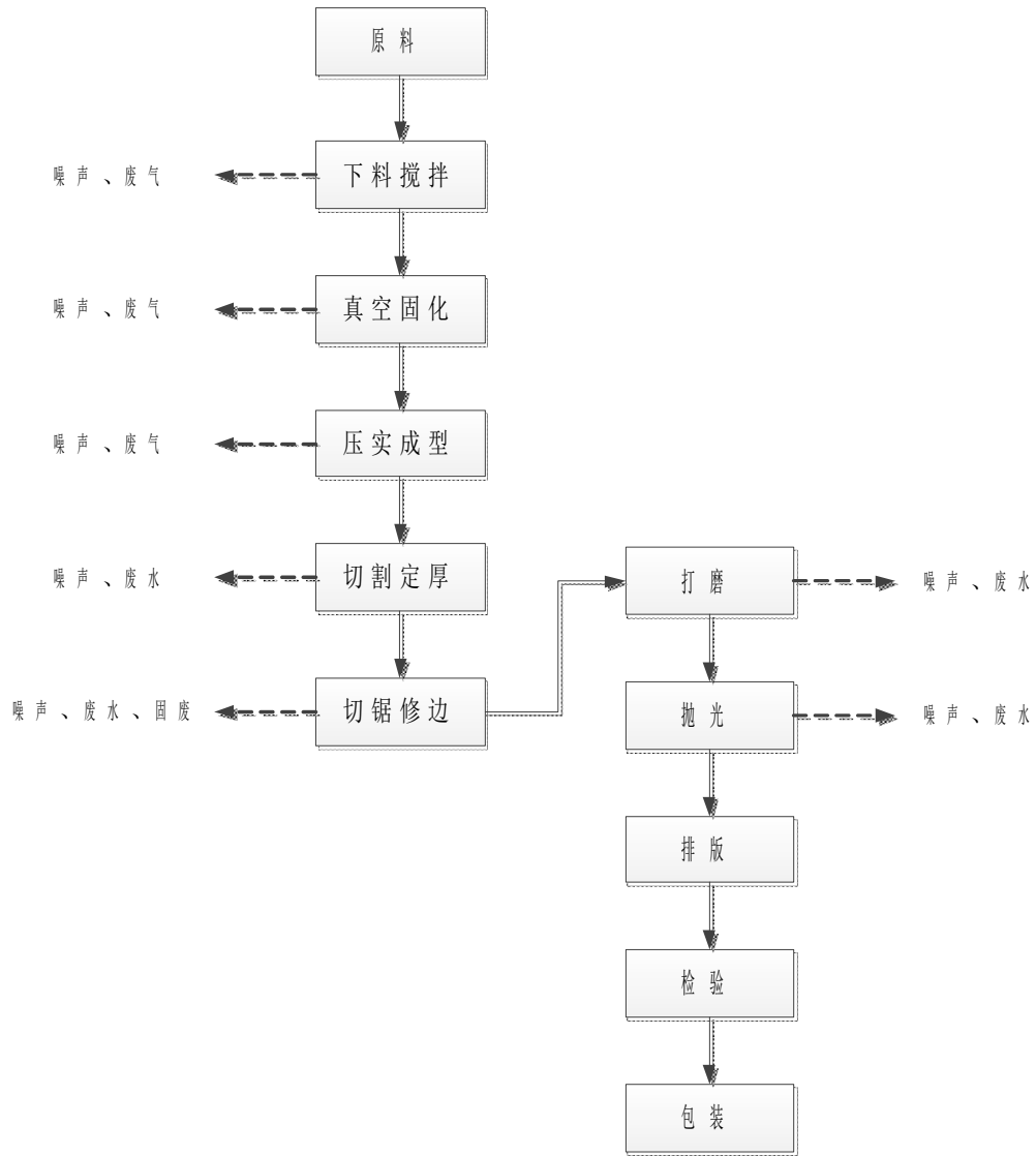
图 4.1-1 人造石材生产工艺
