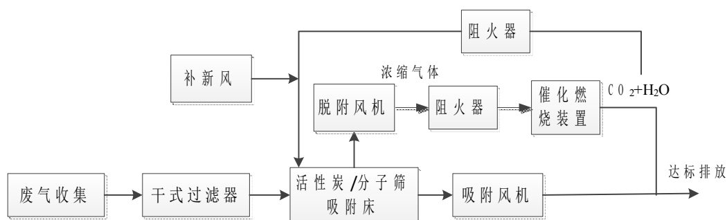
图 5.1-1 “活性炭/分子筛转轮吸附浓缩-催化燃烧”工艺流程图
