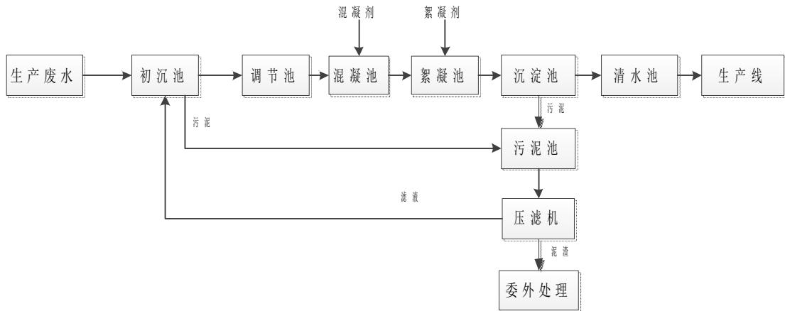
图 5.2-1 生产废水处理工艺流程图
