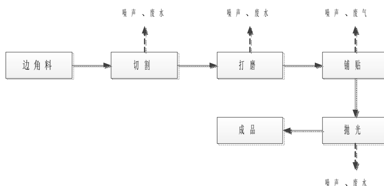
图 4.3-1 人造马赛克生产工艺
