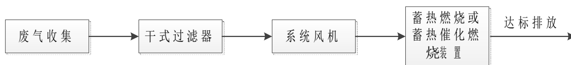
图 5.1-2 “蓄热燃烧或蓄热催化燃烧”工艺流程图
