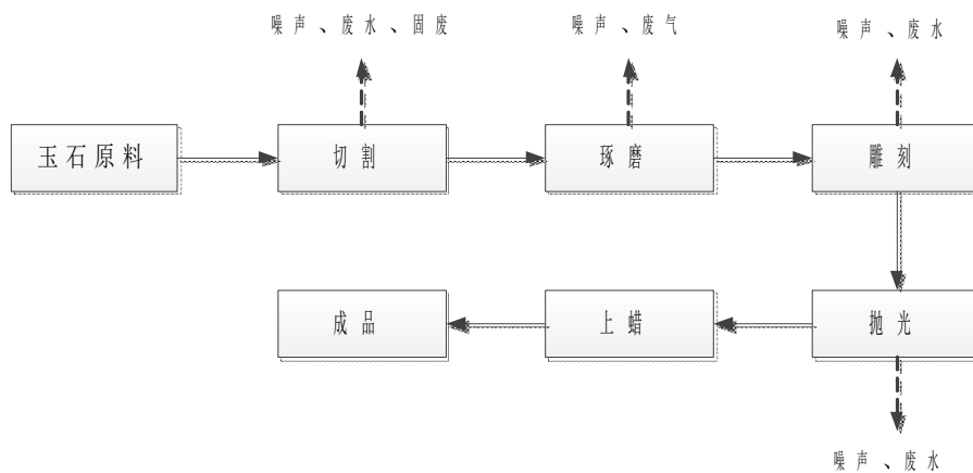
图 4.3-3 玉石加工工艺
