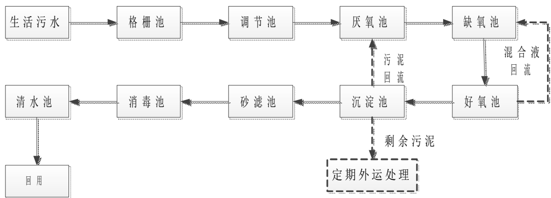
图 5.2-3 生活污水回用工艺流程图
